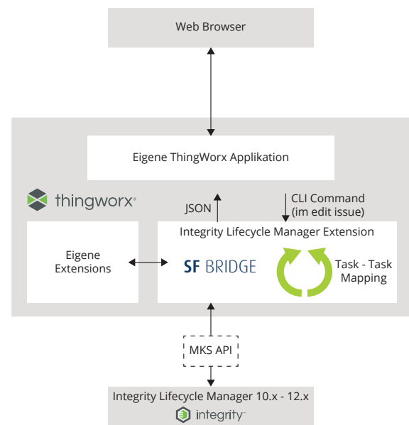
ThingWorx-Architektur mit SF Bridge für PTC ILM & ThingWorx
