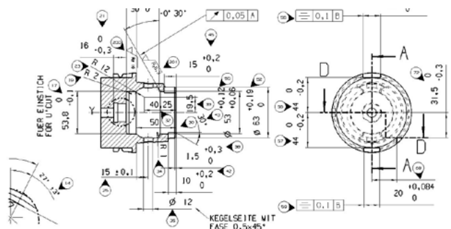
Zeichnung mit Merkmalsnummern
